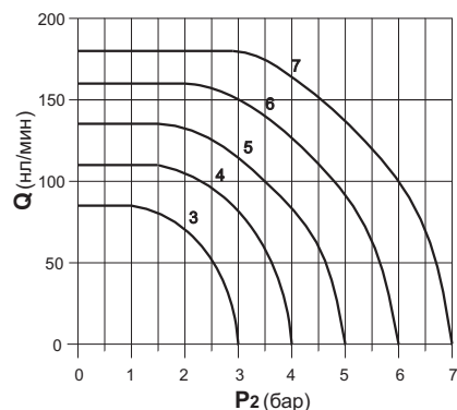
Серия 104, присоединение трубки \varnothing 4 мм
