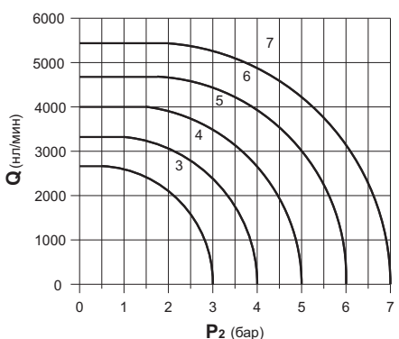
Серия 212, присоединение G1/2" исполнения - 5/3
