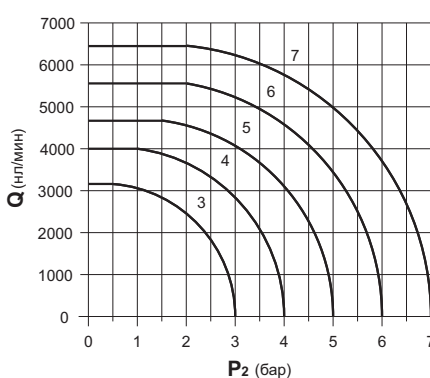
Серия 212, присоединение G1/2" исполнения - 3/2 и 5/2
