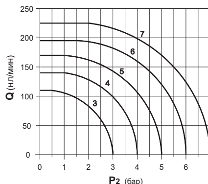
Серия 105, присоединение M5
