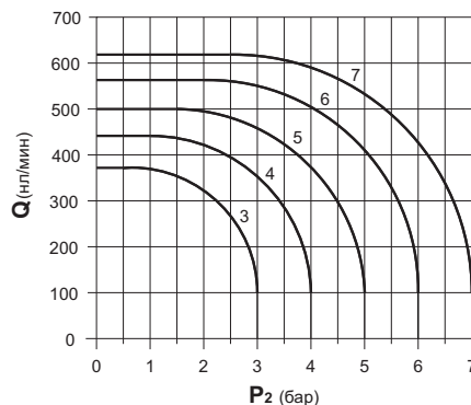
Серия 228, присоединение G1/8" исполнения - 5/3
